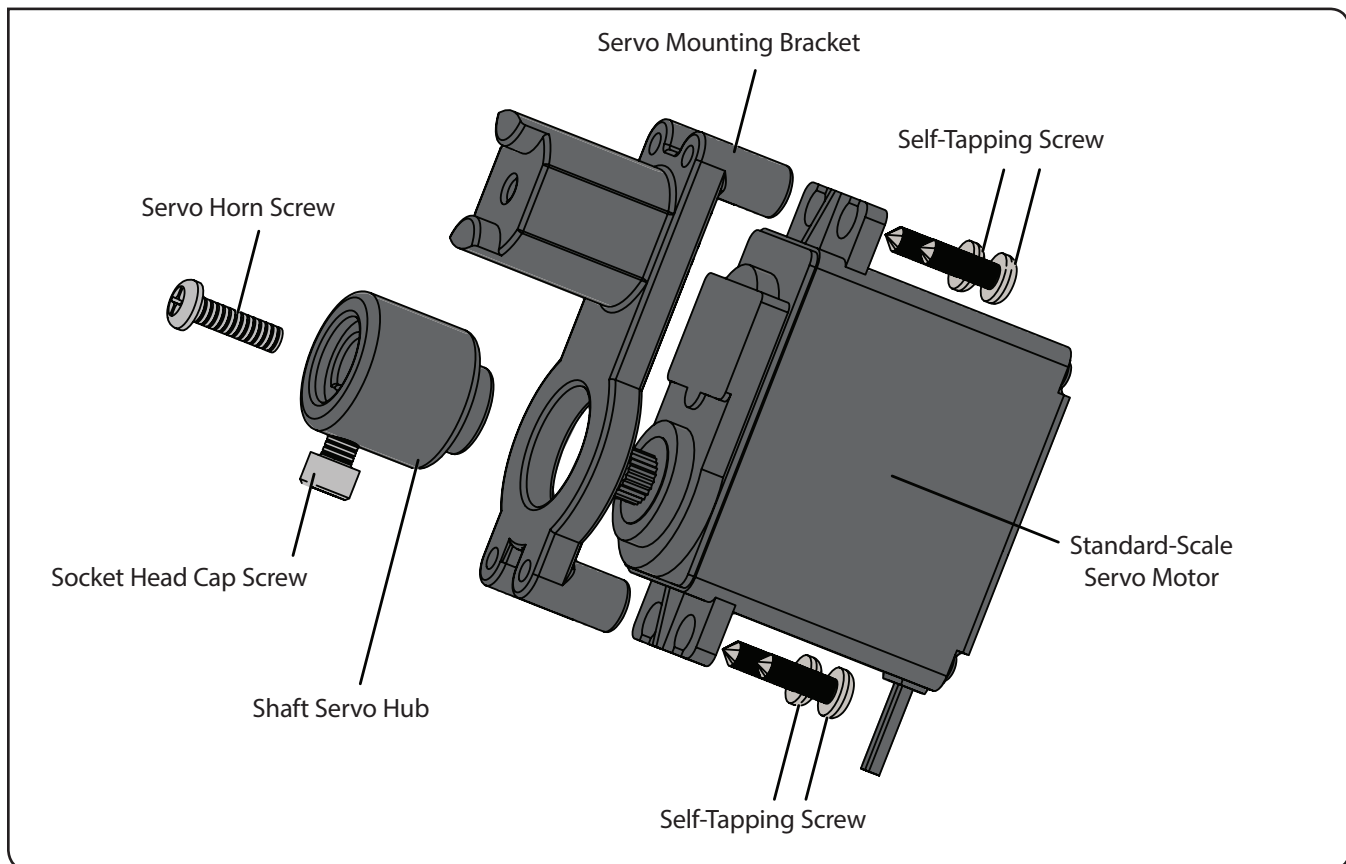
1x Standard-Scale Servo Motor 40538
