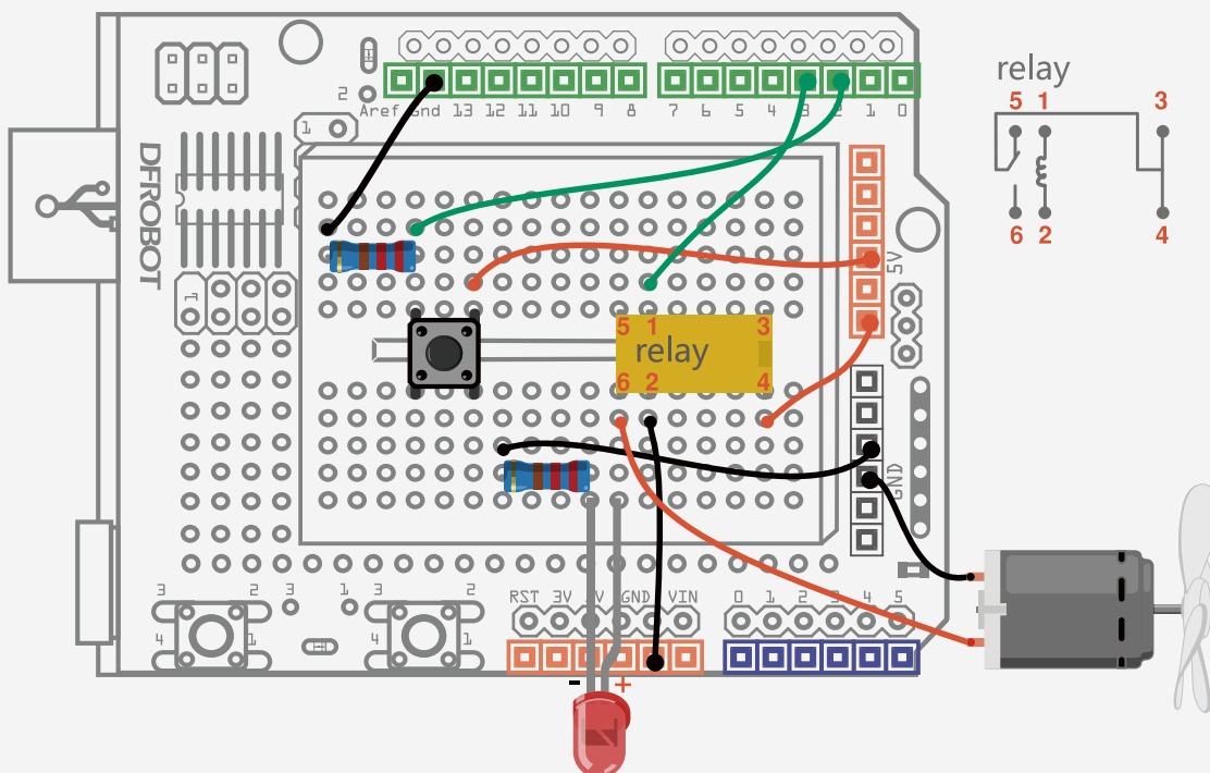
Fig. 13-1 DIY Fan Circuit Diagram
