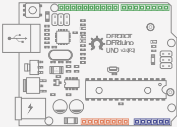
DFRduino UNO R3 x1
