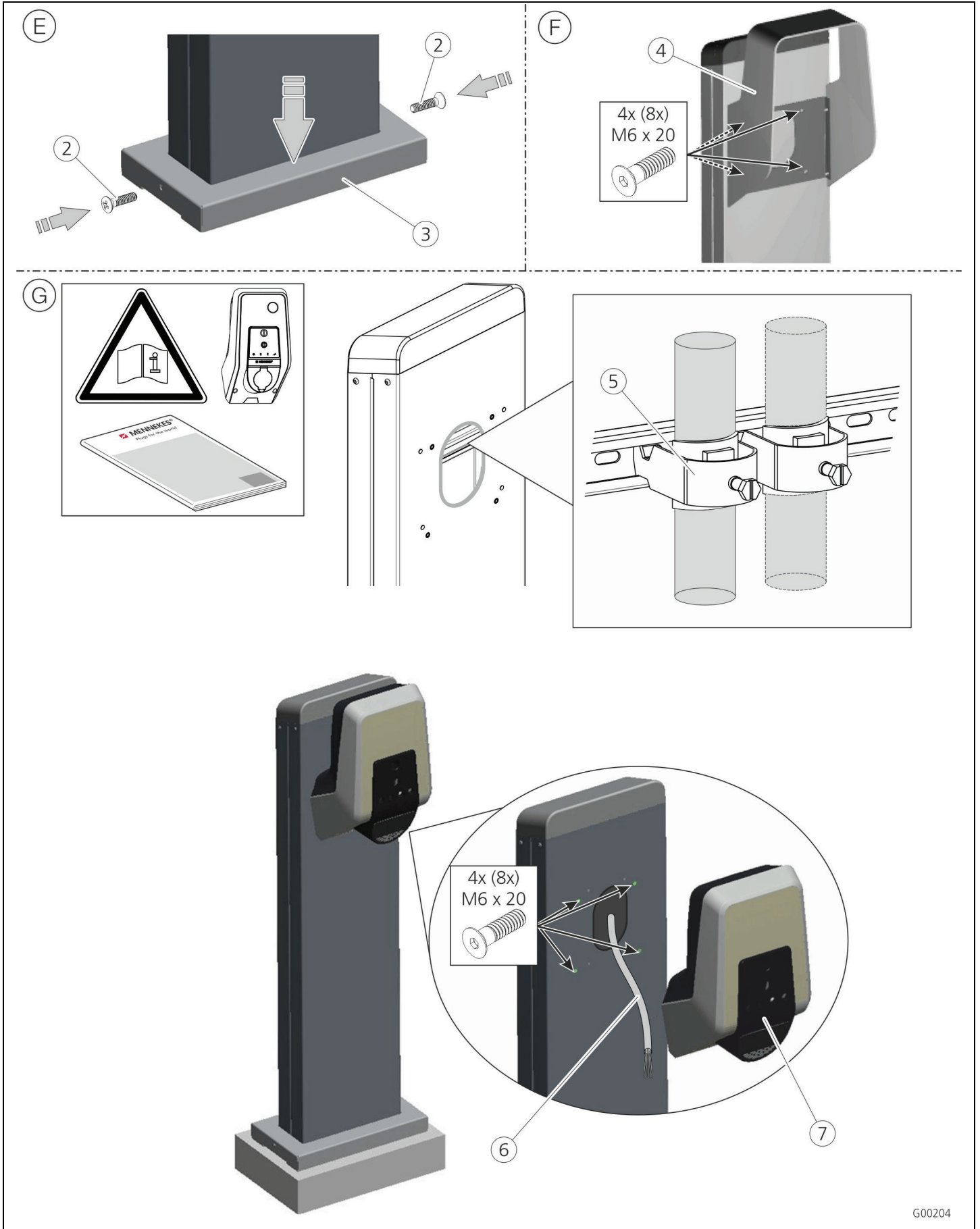
Abb. 3: Montage Ladestation
