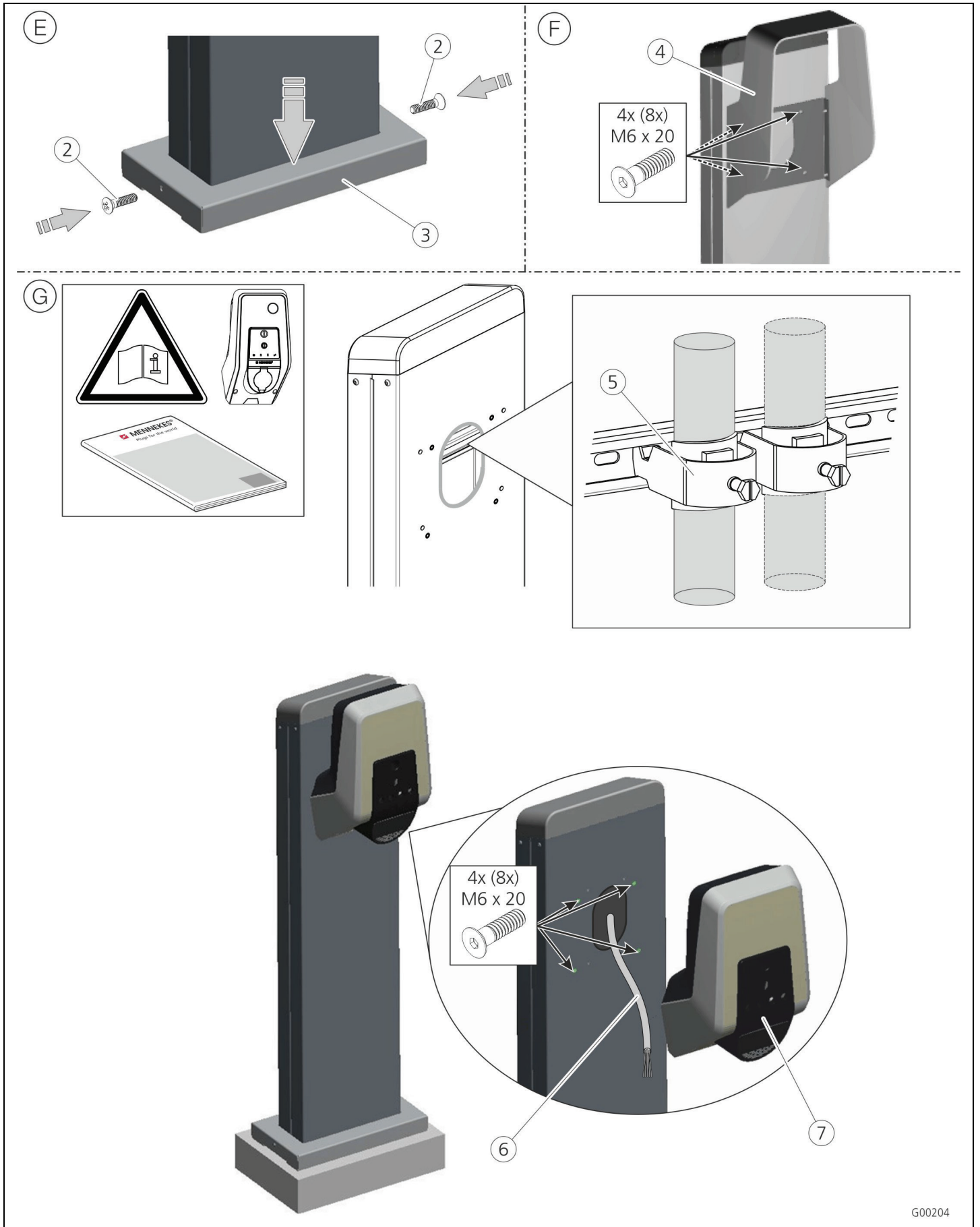
Afb. 3: Montage laadstation
